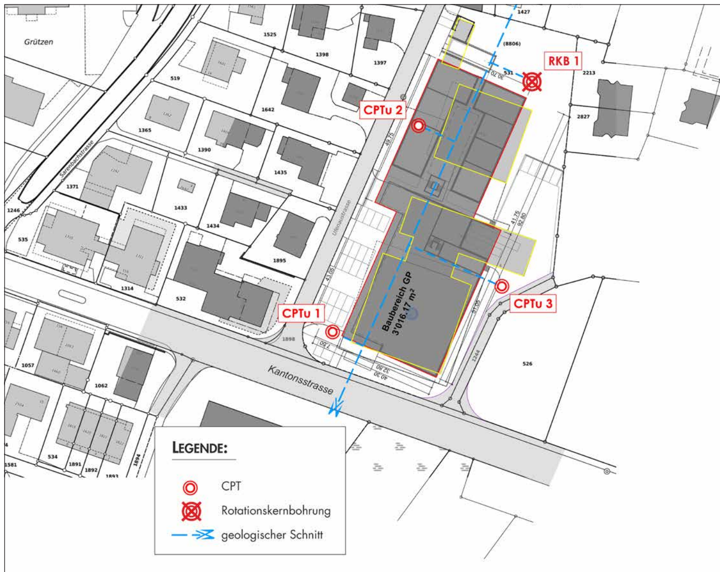
Baugrundsondierung – Situation 1 : 1000
