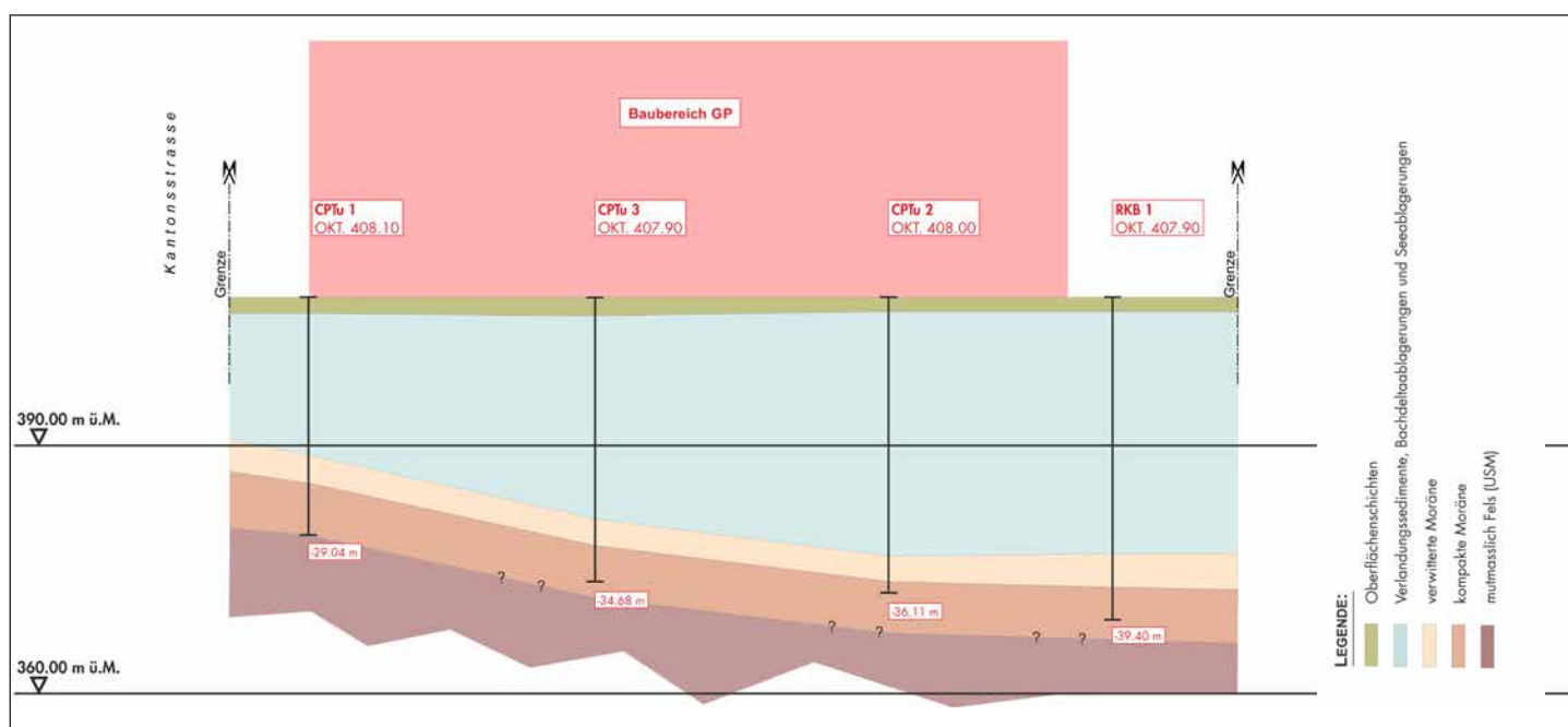
Baugrundsondierung – Schnitt 1 : 500
